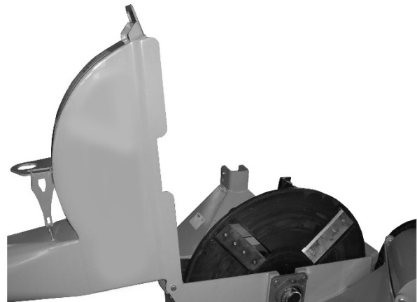
Fig. 47 Afkasthætte
