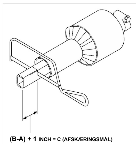
Fig. 34 AFSKÆRINGSMÅL
