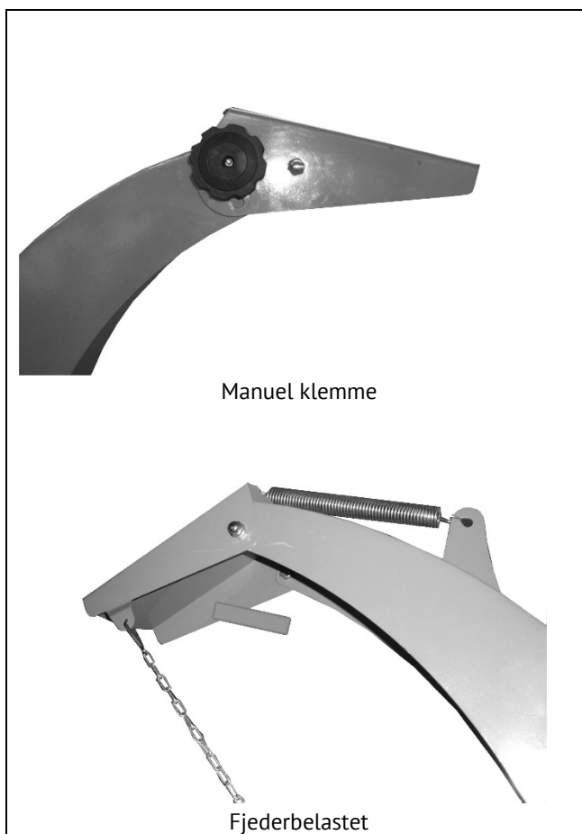
Fig. 37 DEFLEKTOR-POSITION
