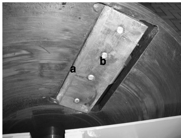
Fig. 41 Rotorblade
