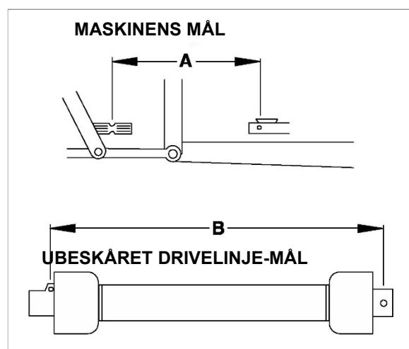
Fig. 33 DRIVELINJE-MÅL
